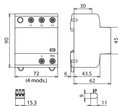
Beépítési méretek
