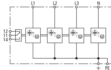
Kapcsolási rajz
