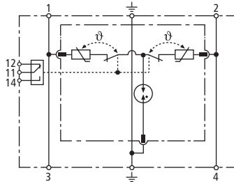
Kapcsolási rajz
