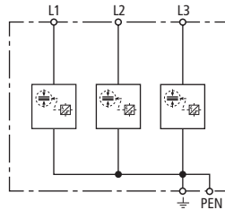
Kapcsolási rajz
