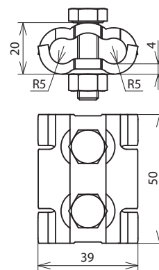
Beépítési méretek
