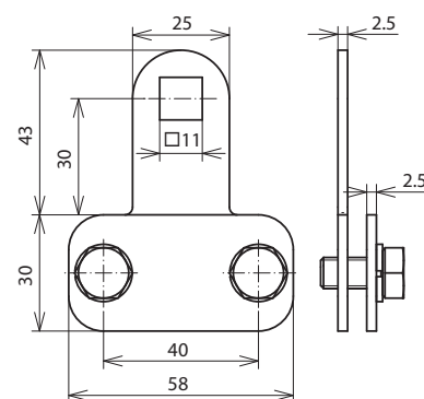
Beépítési méretek
