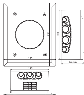
Beépítési méretek
