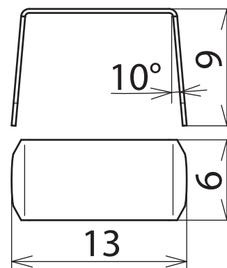
Beépítési méretek
