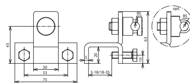
Beépítési méretek
