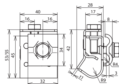
Beépítési méretek
