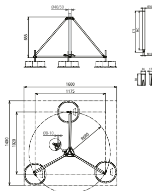
Beépítési méretek
