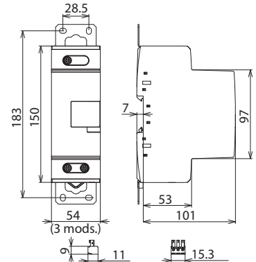
Beépítési méretek
