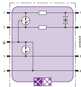
Kapcsolási rajz
