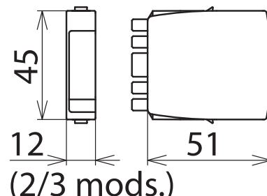
Beépítési méretek
