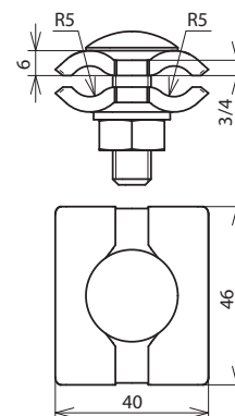
Beépítési méretek
