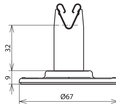
Beépítési méretek
