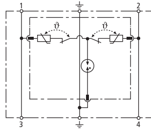
Kapcsolási rajz
