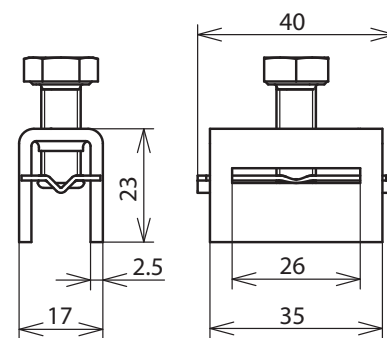
Beépítési méretek
