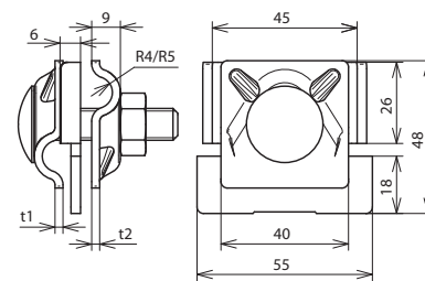
Beépítési méretek
