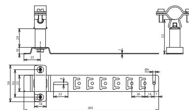
Beépítési méretek
