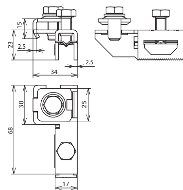
Beépítési méretek
