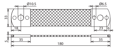
Beépítési méretek
