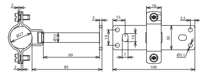
Beépítési méretek
