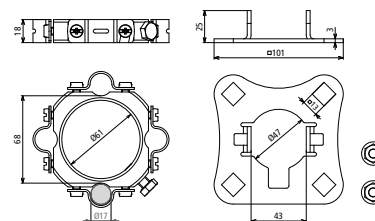
Beépítési méretek
