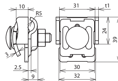
Beépítési méretek
