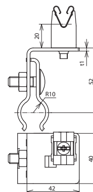
Beépítési méretek
