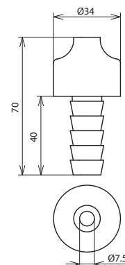
Beépítési méretek
