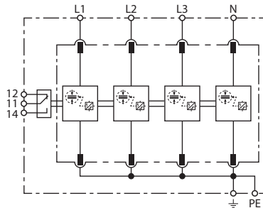
Kapcsolási rajz
