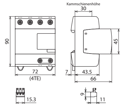
Beépítési méretek
