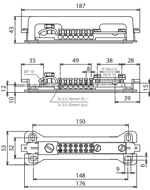
Beépítési méretek
