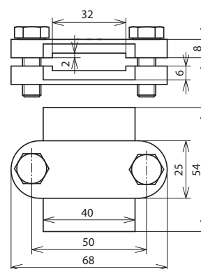
Beépítési méretek
