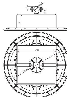
Beépítési méretek
