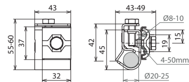
Beépítési méretek
